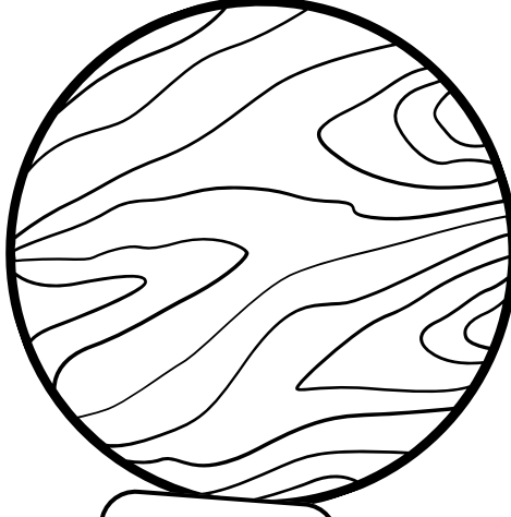
URANÜS
