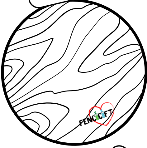
NEPTÜN
