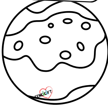
MARS
