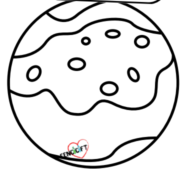
MARS
