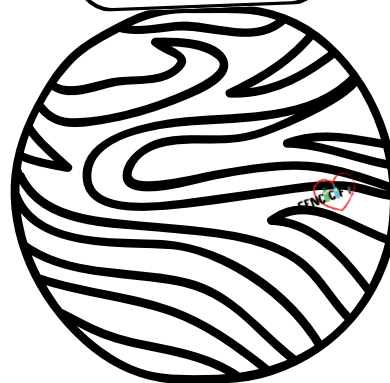
VENÜS
