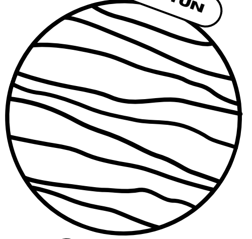
NEPTÜN
